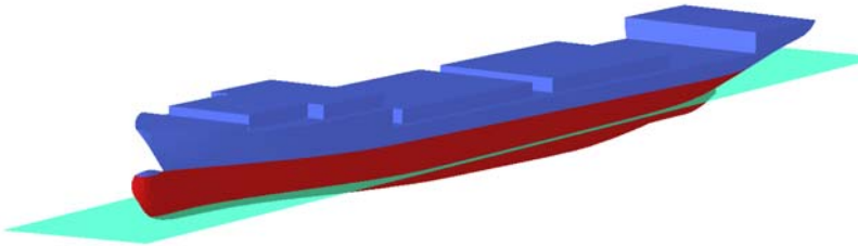
Fig.4 Locopias 3D uitvoer schip inclusief waterlijn
